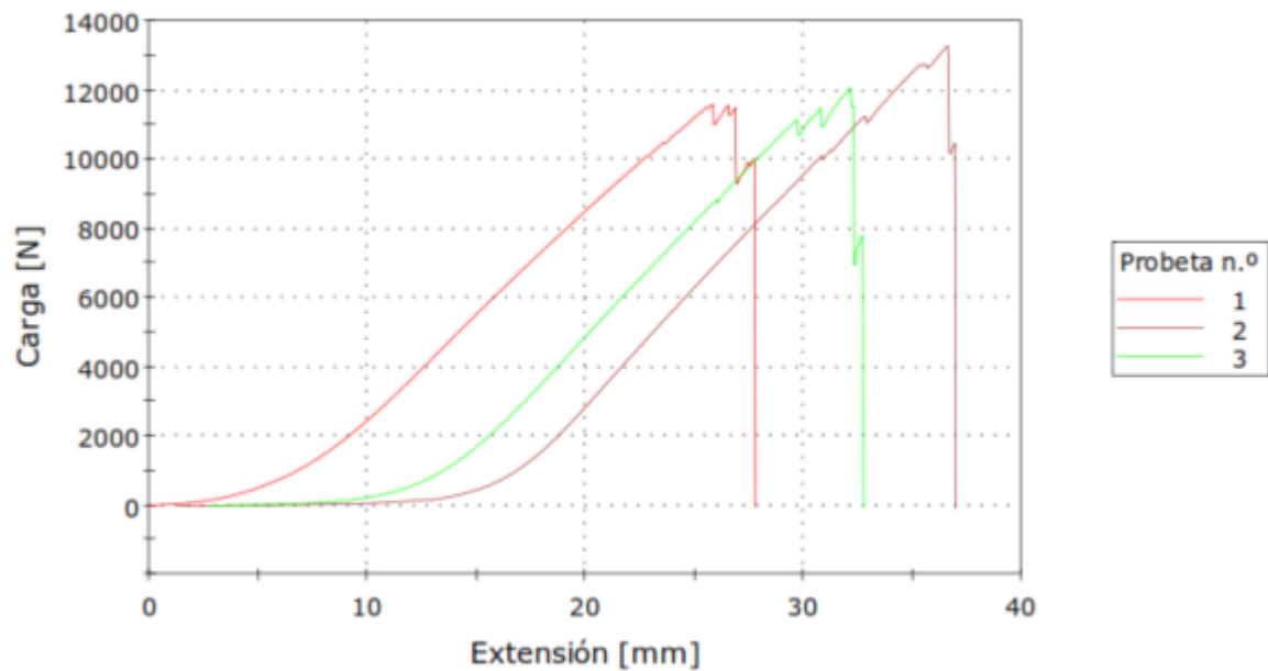
Grafica de carga vs extensión de la cinta
